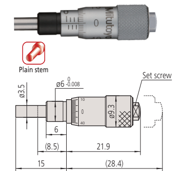
148-201-10 Mass: 10 g
